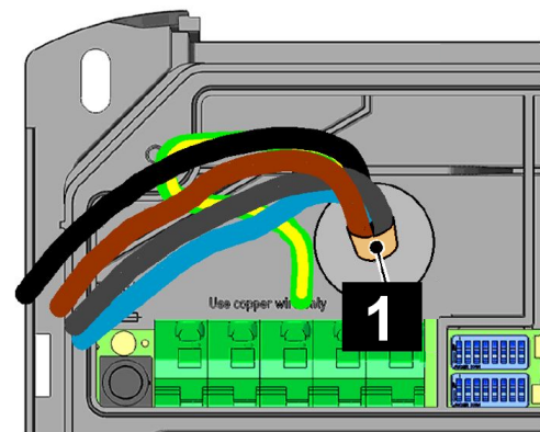
Embout double membrane (montage de câble encastré)
