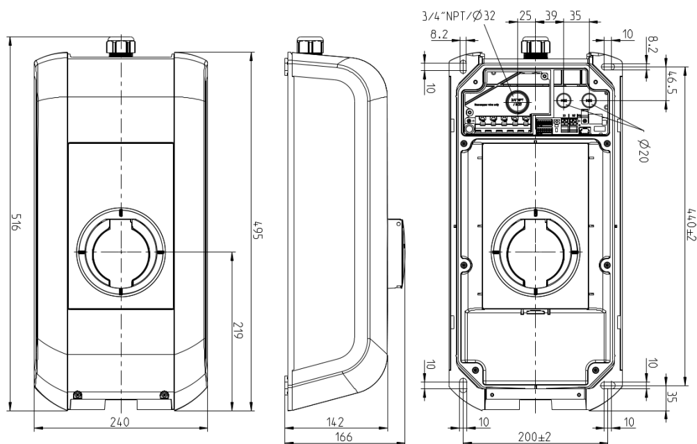
Fig. 12-20: Dimensions en millimètres
